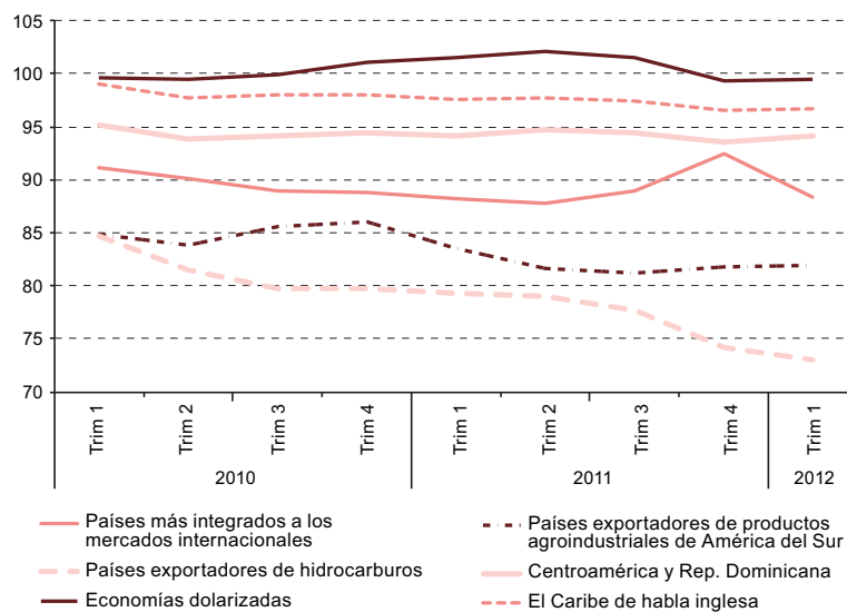
Gráfico 19 AMÉRICA LATINA Y EL CARIBE: TIPO DE CAMBIO REAL EFECTIVO EXTRARRREGIONAL (Base 2005=100)
