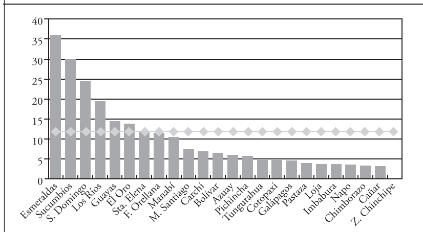
Gráfico 1: Tasa de homicidios por cada 100 mil habitantes a nivel provincial (Ene - Jul 2009)
